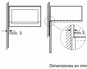
Microondas Montaje en esquina
