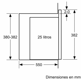
Microondas Montaje en esquina
